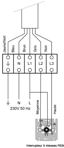
Interrupteur 3 vitesses RS3
